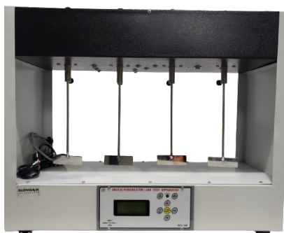
JAR TEST APPARATUS
